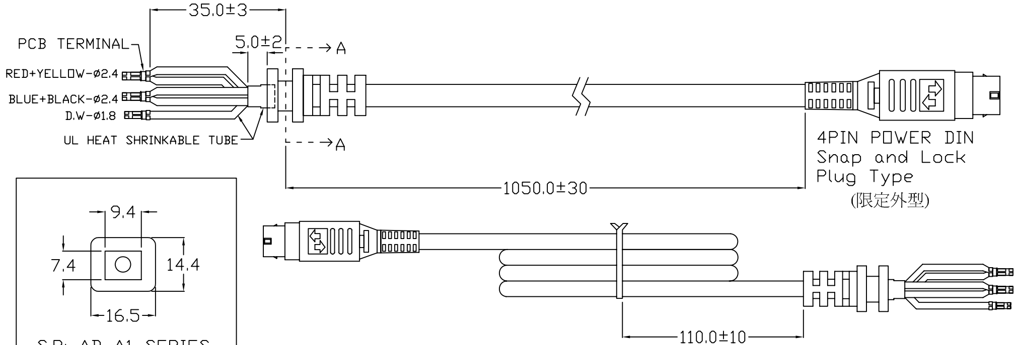
4P POWER DIN FRONT VIEW
