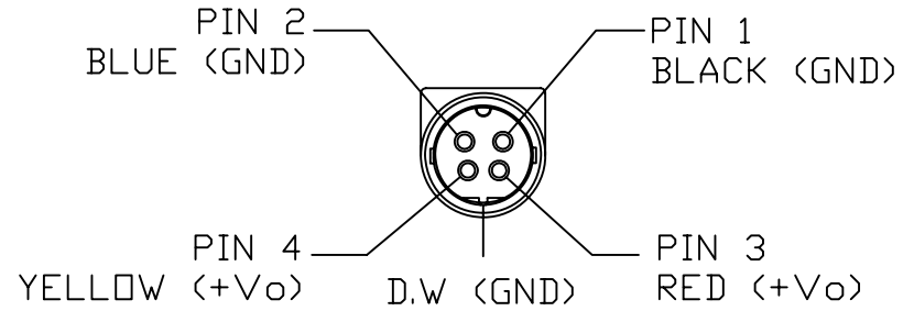
4P POWER DIN FRONT VIEW
